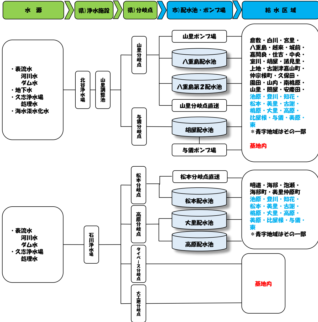
図1. 給水系統概略図
