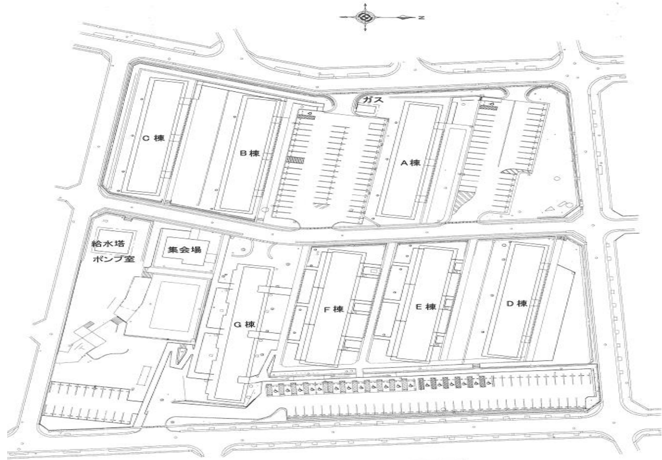
登川市営住宅配置図
