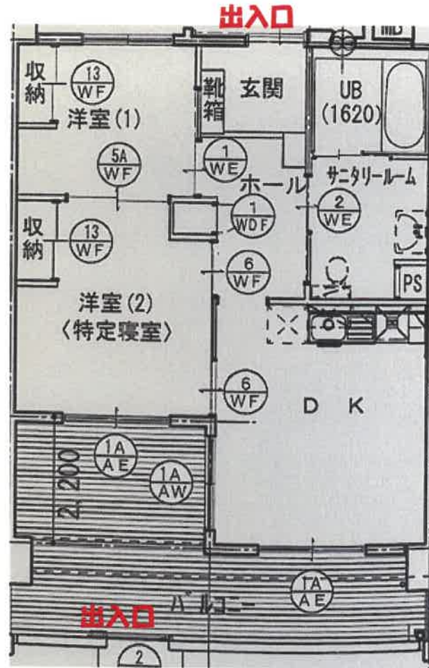
2DK(車椅子住宅) ※下肢障害2級以上の方がいる世帯
