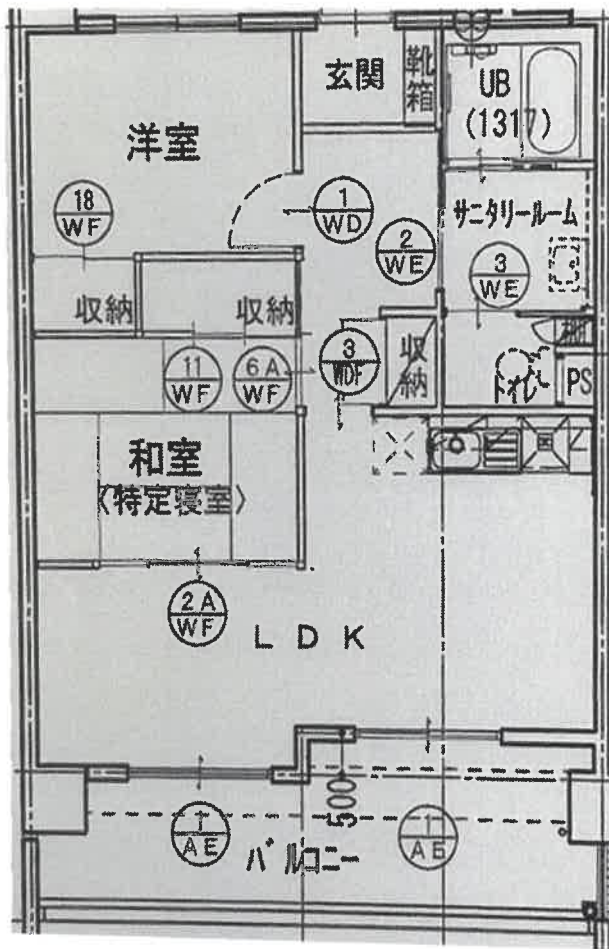
2LDK(一般住宅)
