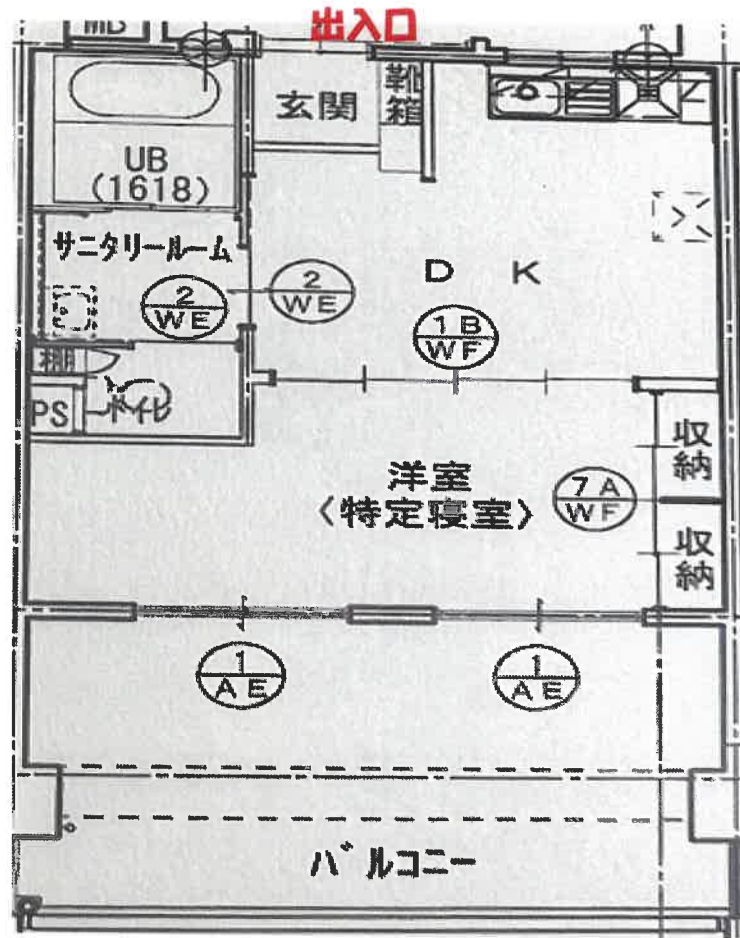
1DK(高齢者住宅)※単身可
