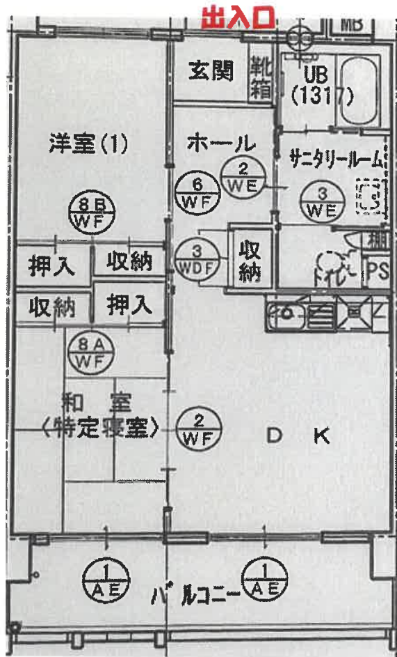
2DK(一般住宅)
